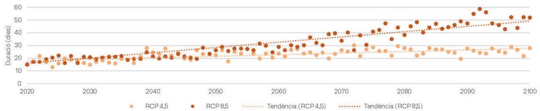
Duració màxima de les onades de calor Escenaris RCP 4,5 i 8,5 - Comarques de la Plana
